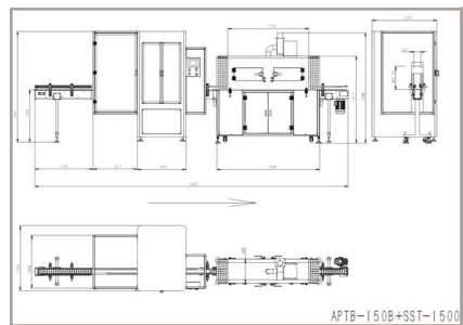
APTB-150B+SST-1500
